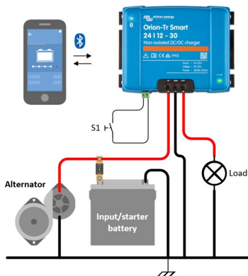
Abbildung 1: Typischer Verbindungsaufbau als DC-DC-Wandler
