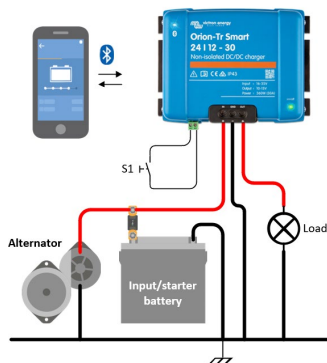
Obrázek 1: Typické nastavení připojení v režimu měniče DC-DC
